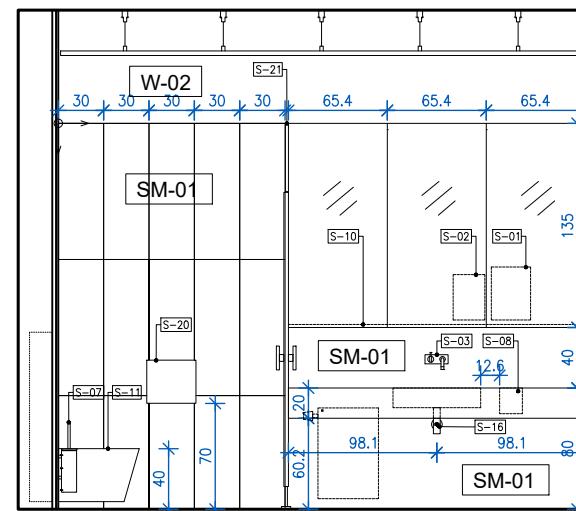
WIDOK 2
