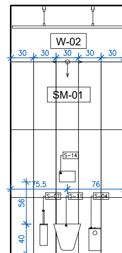
WIDOK 5
