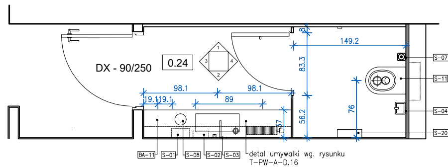
RZUT
