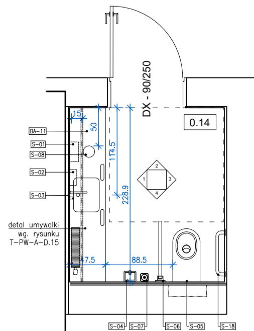
RZUT
