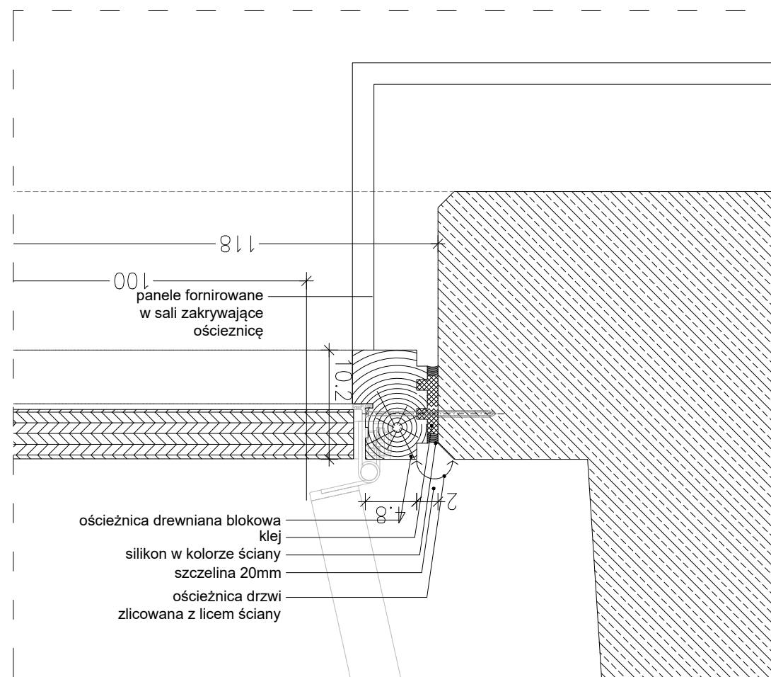
DETAL OSADZENIA DRZWI W ŚCIANIE ŻELBETOWEJ. UWAGA – ANALOGICZNIE WSZYSTKIE DRZWI NA POZ. – 1
